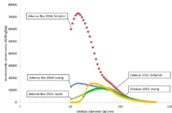
Abbildung 5: Die Teilchengrößenverteilung im Feinstaub in Cabauw und im Amsterdamse Bos.
