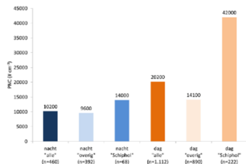
Abbildung 3: Stündliche Durchschnittswerte für PNC im Amsterdame Bos von März bis Mai 2014 bei Tagstunden (,dag') und Nachtstunden (,nacht') (n), bei allen Windrichtungen (,alle'), bei Wind aus Richtung Schiphol: 240-270° (,Schiphol') sowie bei Wind aus anderen Windrichtungen (,overig').
