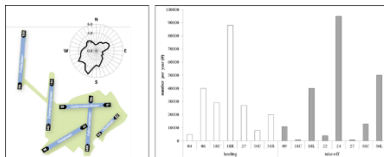
Abbildung 1: Links: Die Start- und Landebahnen mit zugehöriger Bezeichnung sowie die Windrichtungsverteilung (in Prozent) im Jahr 2012. Rechts: Die Anzahl landender und startender Flugzeuge pro Start- und Landebahn auf Schiphol im Jahr 2012.
