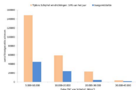
Abbildung 7: Belastung der Bevölkerung durch von Schiphol ausgehendes zusätzliches PNC (Partikelzahl/cm 3 ) bei Wind aus Richtung Schiphol (rosa) und im Jahresdurchschnitt (blau) im Jahr 2012.
