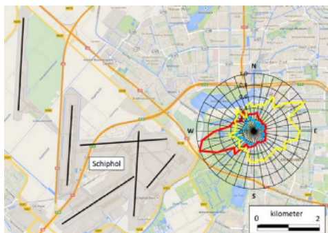
Abbildung 2: Standardisierte stündliche Mittelwerte von PNC und EC im Amsterdame Bos bei verschiedenen Windrichtungen: für EC in Gelb für alle Stunden der Messperiode (n=1 486), für PNC in Blau für Nachtstunden (n= 460) und in Rot für Stunden zur Tageszeit (n= 1 112).
