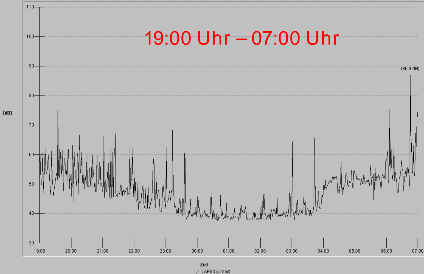
Pegel-Zeitverlauf (LAP03) am 22.05.2012
